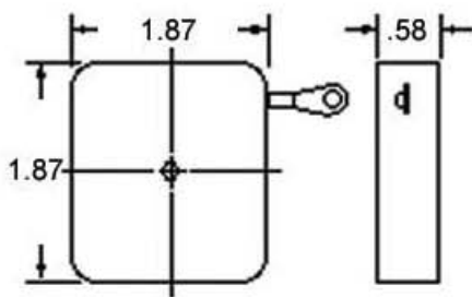
ENCLOSED REEL (ER)
